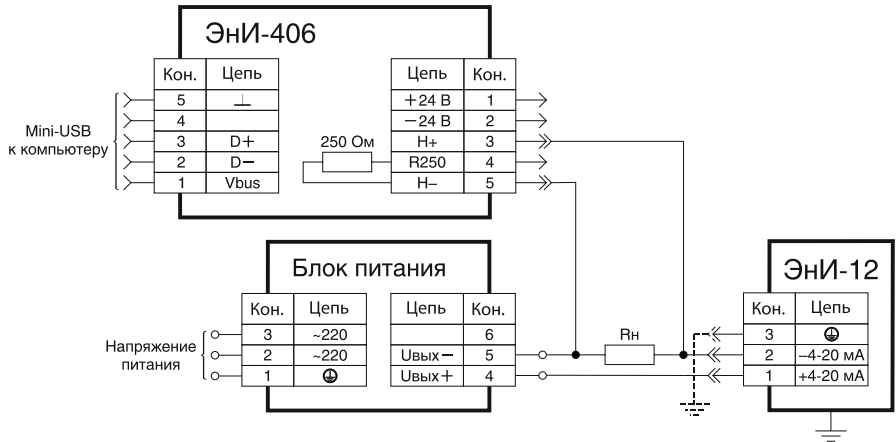
Рисунок В.1 — Подключение датчика ЭНИ-12
