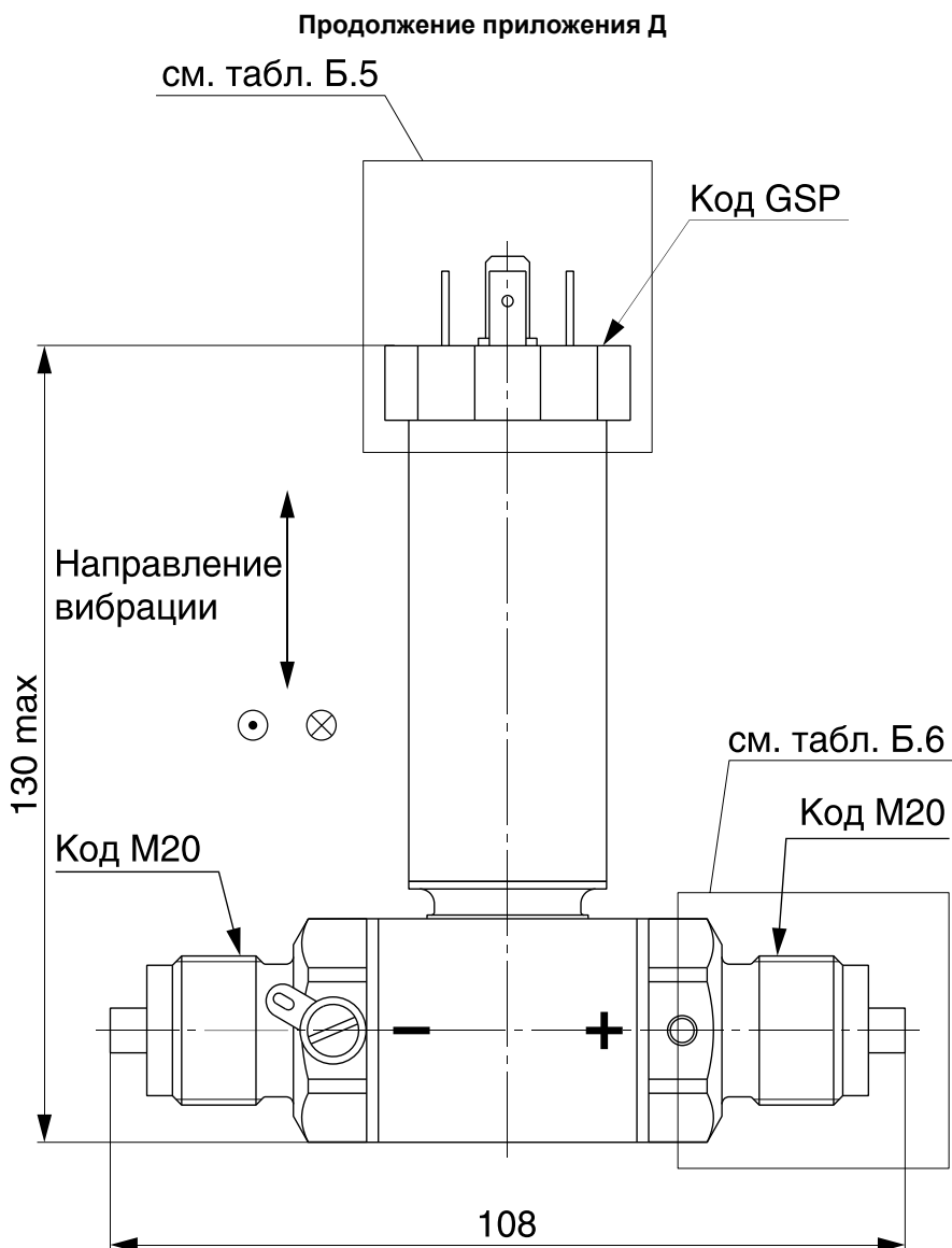
Рисунок Д.5 — Габаритные и присоединительные размеры датчика ЭНИ-12Н моделей ДД
