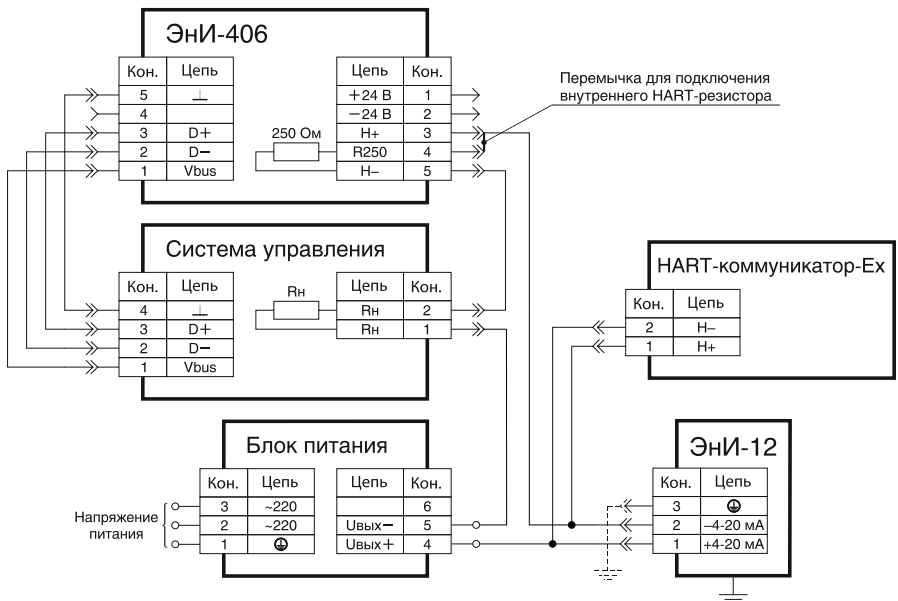
Рисунок В.2 — Вариант включения датчика с HART-модемом
