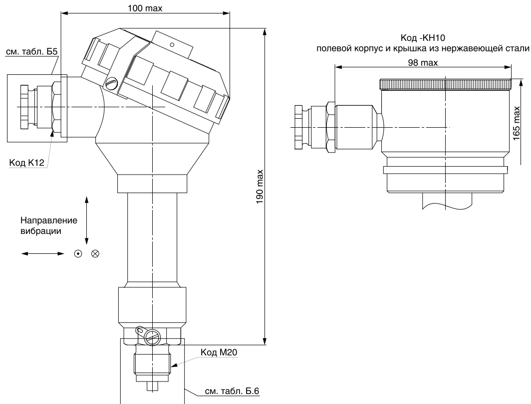
Рисунок Д.4 — Габаритные и присоединительные размеры датчика ЭНИ-12HS моделей ДИ, ДА, ДИВ, ДВ, только для моделей с индексом «М»
