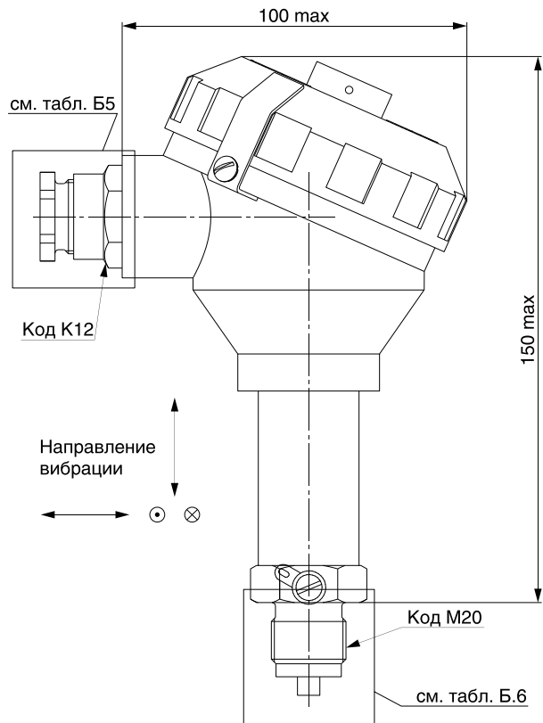
Рисунок Д.3 — Габаритные и присоединительные размеры датчика ЭНИ-12HS моделей ДИ, ДА, ДИВ, ДВ, кроме моделей с индексом «М»
