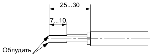
Рисунок 2.1 — Разделка кабеля
