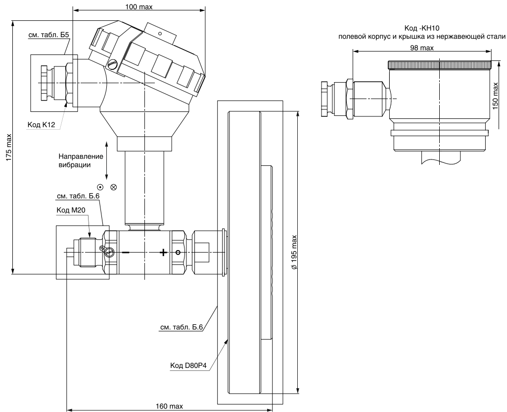
Рисунок Д.8 — Габаритные и присоединительные размеры датчика ЭНИ-12HS моделей ДГ
