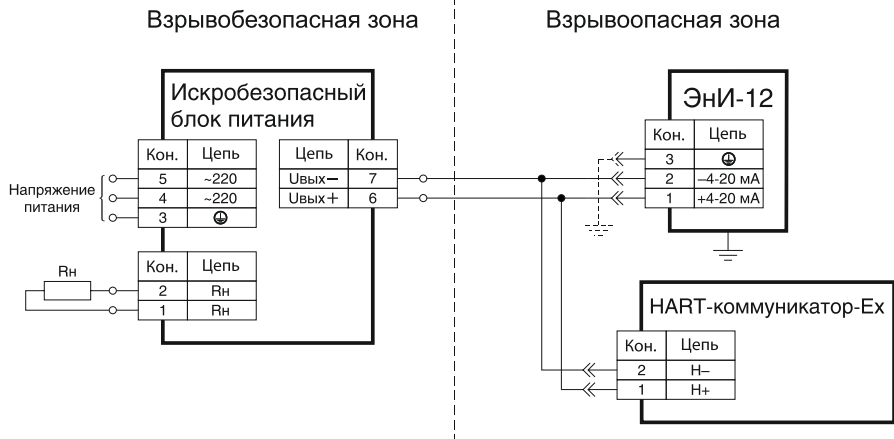
Рисунок В.3 — Вариант включения датчика с блоком искрозащиты
