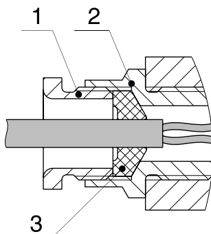
Рисунок 2.1 — Разделка кабеля
